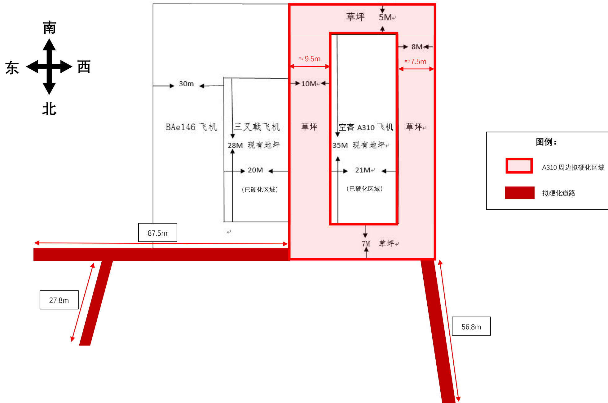
A310 活化利用配套地面硬化示意图
